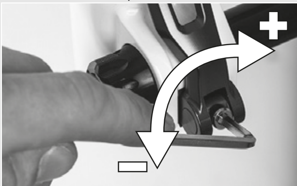
Illustration 33 : Régler la force de serrage de l'attache rapide
