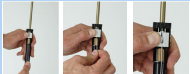
Figura 135: Sgancio del tirante
