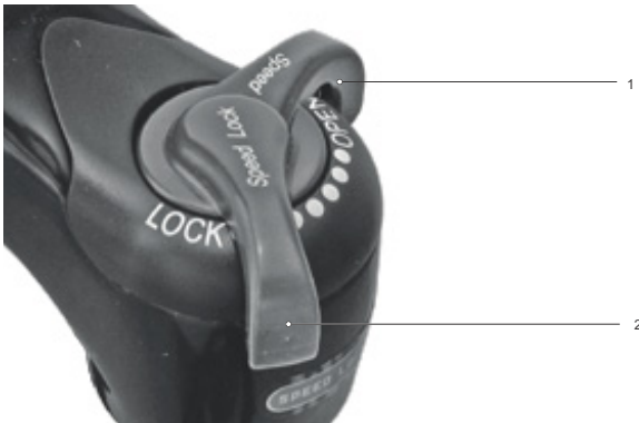
Figura 199: Regolazione più morbida del regolatore dello stadio di compressione
