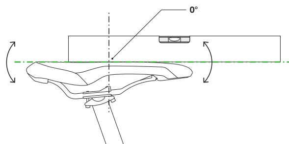
Figura 64: Sella in posizione orizzontale con angolo di inclinazione di 0° del centro della sella
