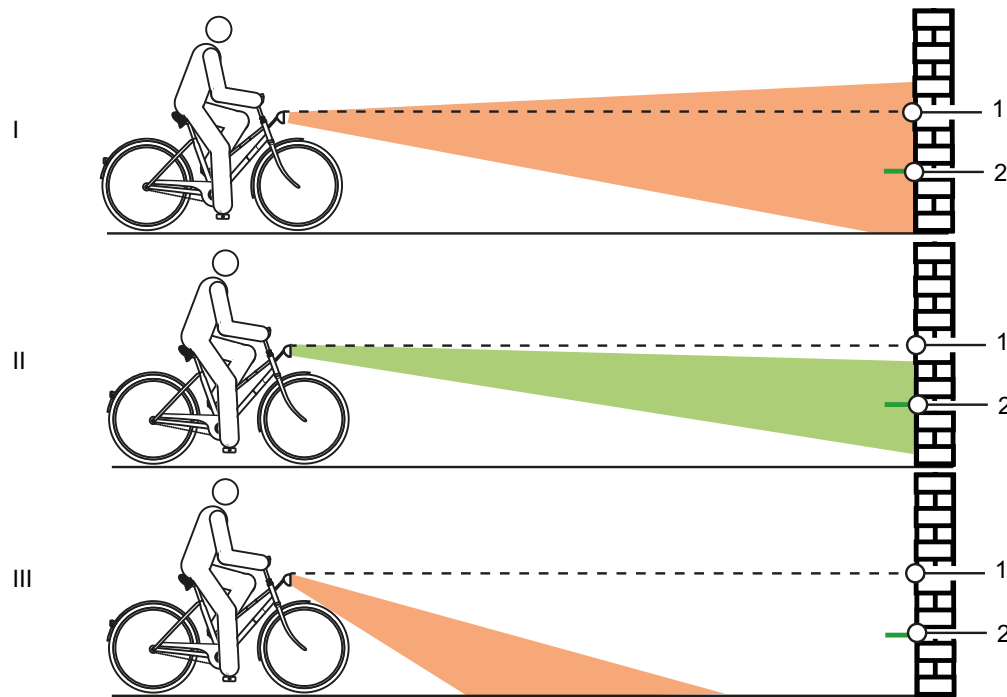
Figura 120: Luce regolata a un'altezza eccessiva (1), correttamente (2) e a un'altezza insufficiente (3)
