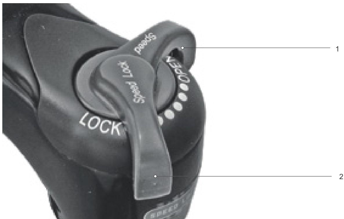
Figura 107: Ammortizzatore a stadi di pressione Suntour in posizione aperta (1) e chiusa (2)
