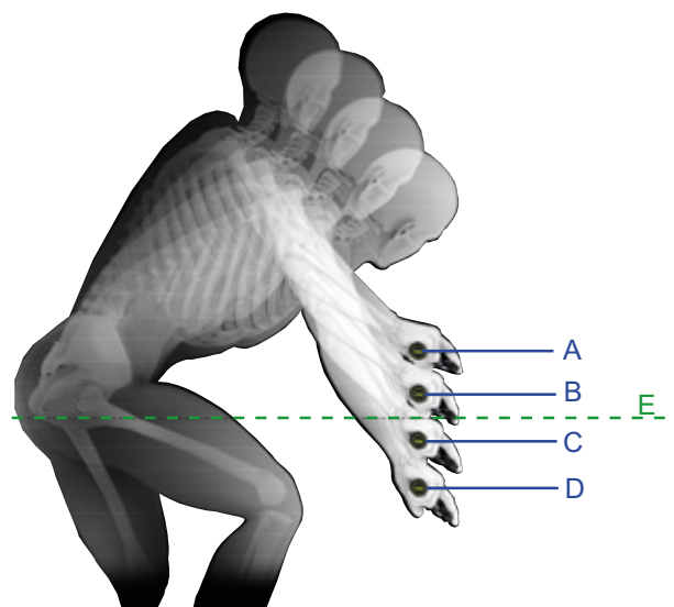
Figura 77: Esempio: 4 altezze diverse del manubrio (A, B, C e D) e altezza della sella (E).
