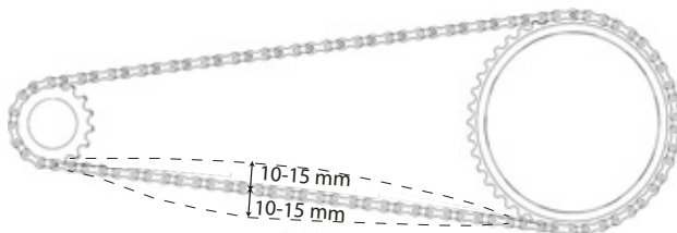
Figura 121: Controllo della tensione della catena
