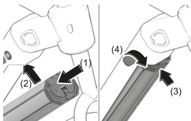
Figura 101: Montaggio della batteria
