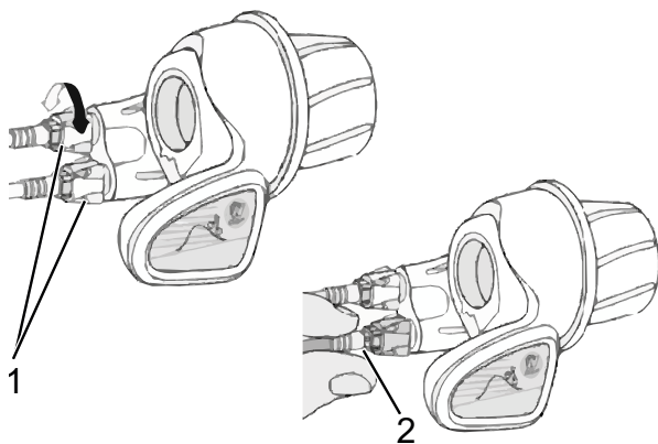
Figura 126: Interruttore a manopola del cambio con boccole di regolazione (1) e gioco della boccola del cambio (2)
