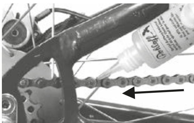
Figura 114: Lubrificazione della catena
