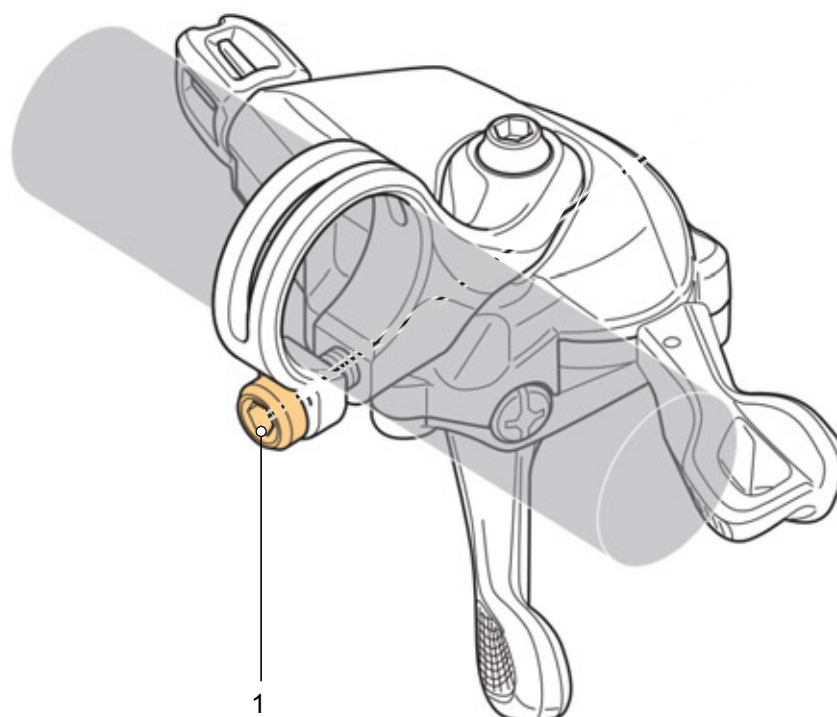
Figura 80: Ubicazione della vite di fissaggio della leva del cambio SHIMANO
