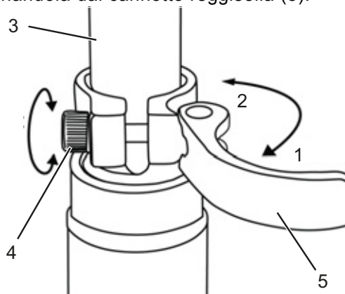
Figura 60: Apertura del bloccaggio rapido del canotto reggisella
