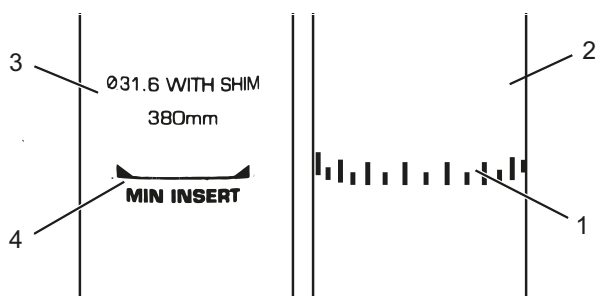
Figura 61: Particolare dei cannotti reggisella, esempi di segno indicante la minima profondità di inserimento
