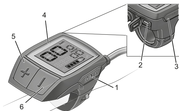
Figura 123: Estructura del ordenador de a bordo BOSCH Purion
